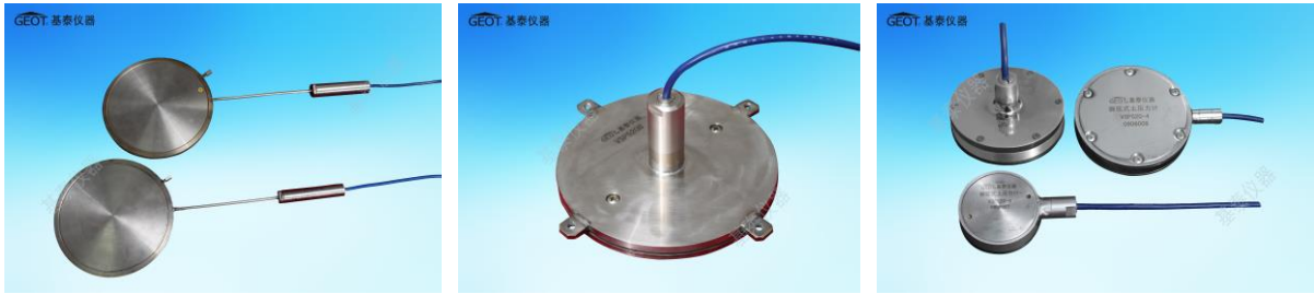
图 1: VSP520A 型土中土压力计 图 2: VSP520B 高精度压力计 图 3: VSP520S 界面式土压力盒
